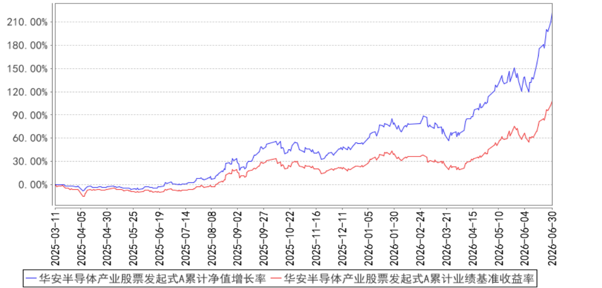
华安半导体产业股票发起式A累计净值增长率与同期业绩比较基准收益率的历史走势对比图
